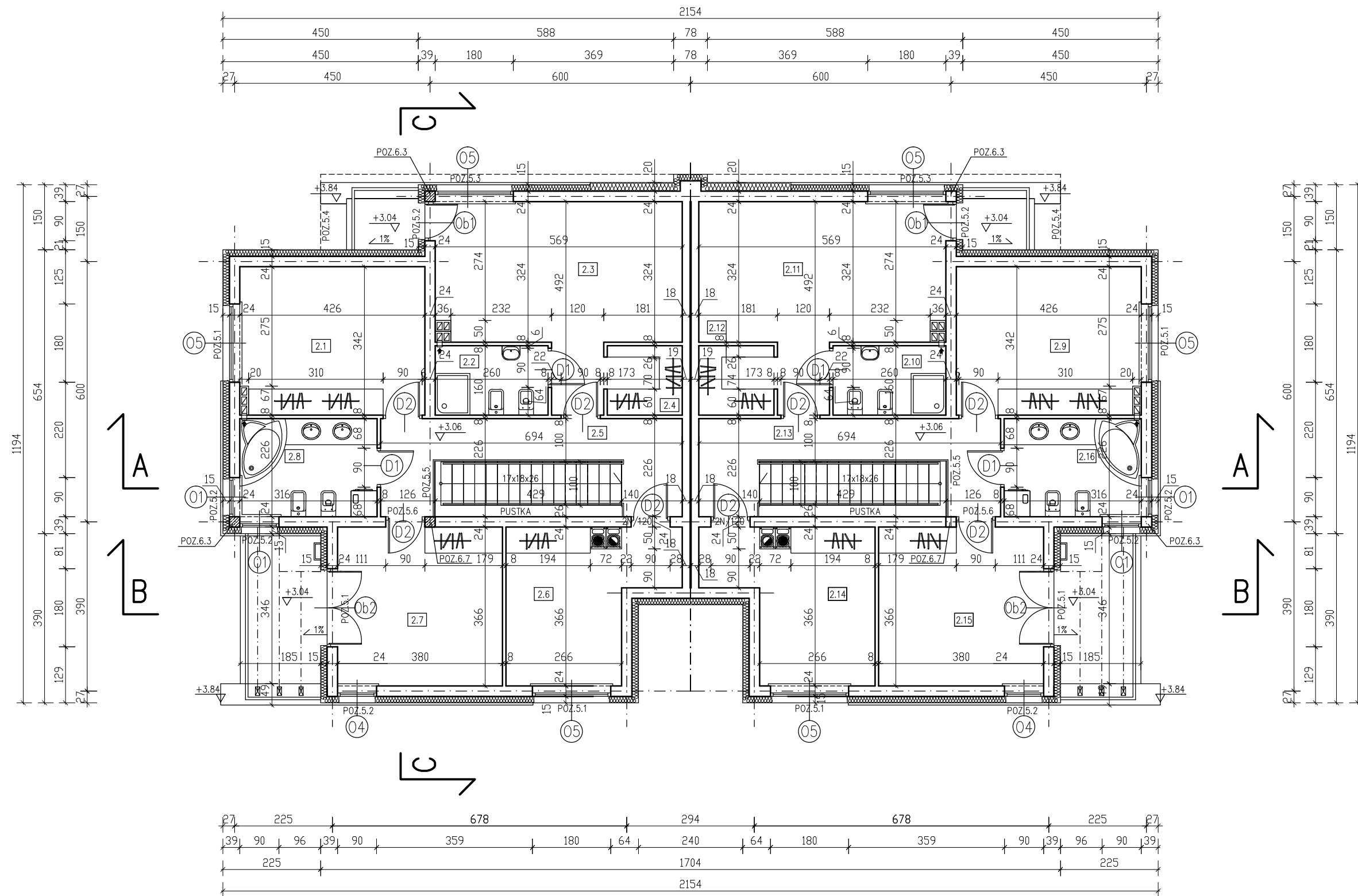
RZUT PIĘTRA 1:100
