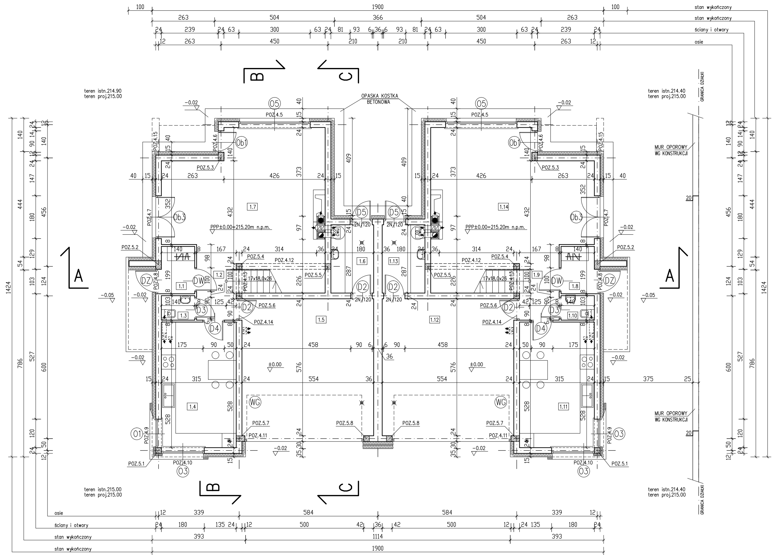
RZUT PARTERU 1:100
