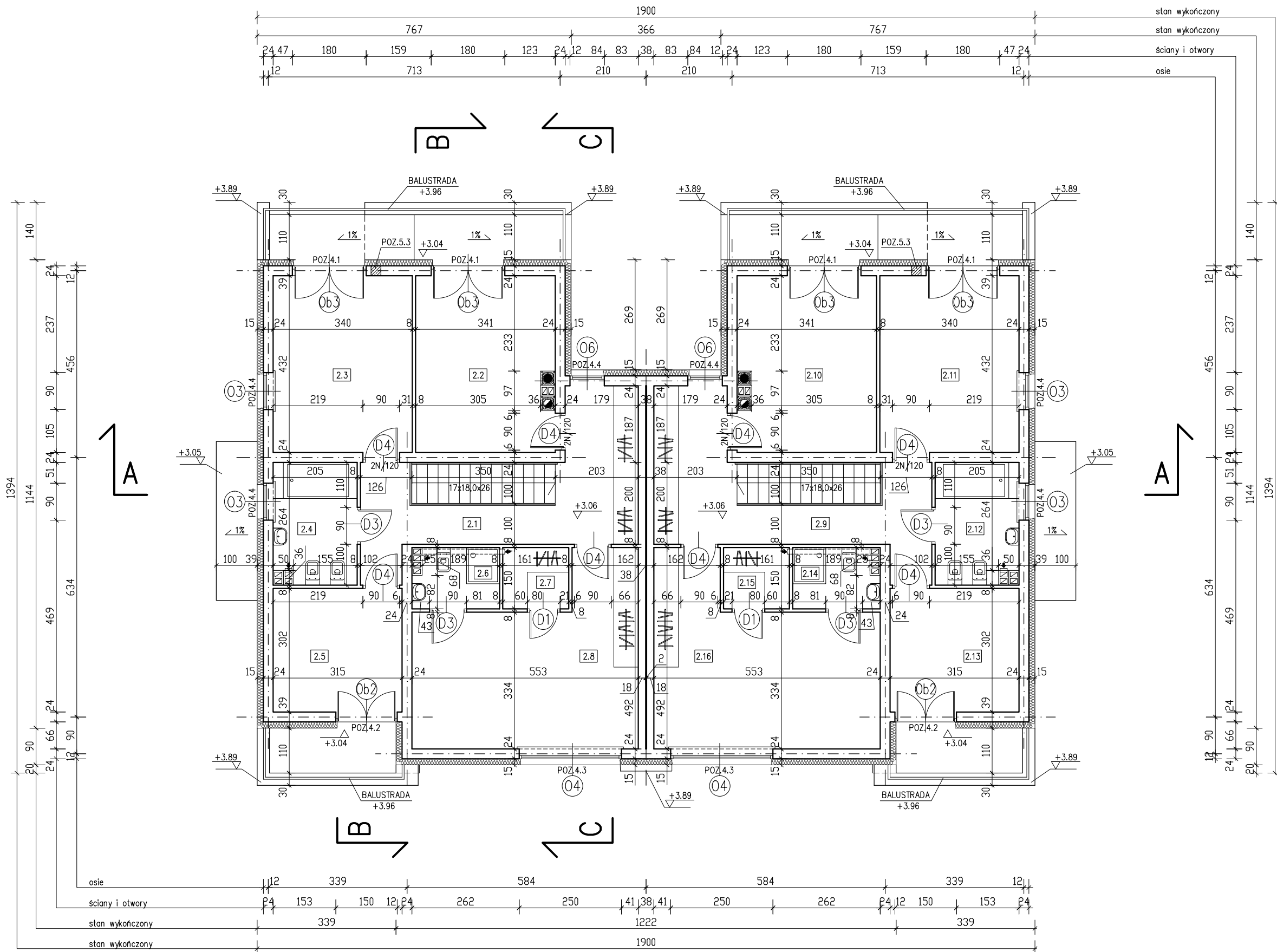
RZUT PIĘTRA 1:100
