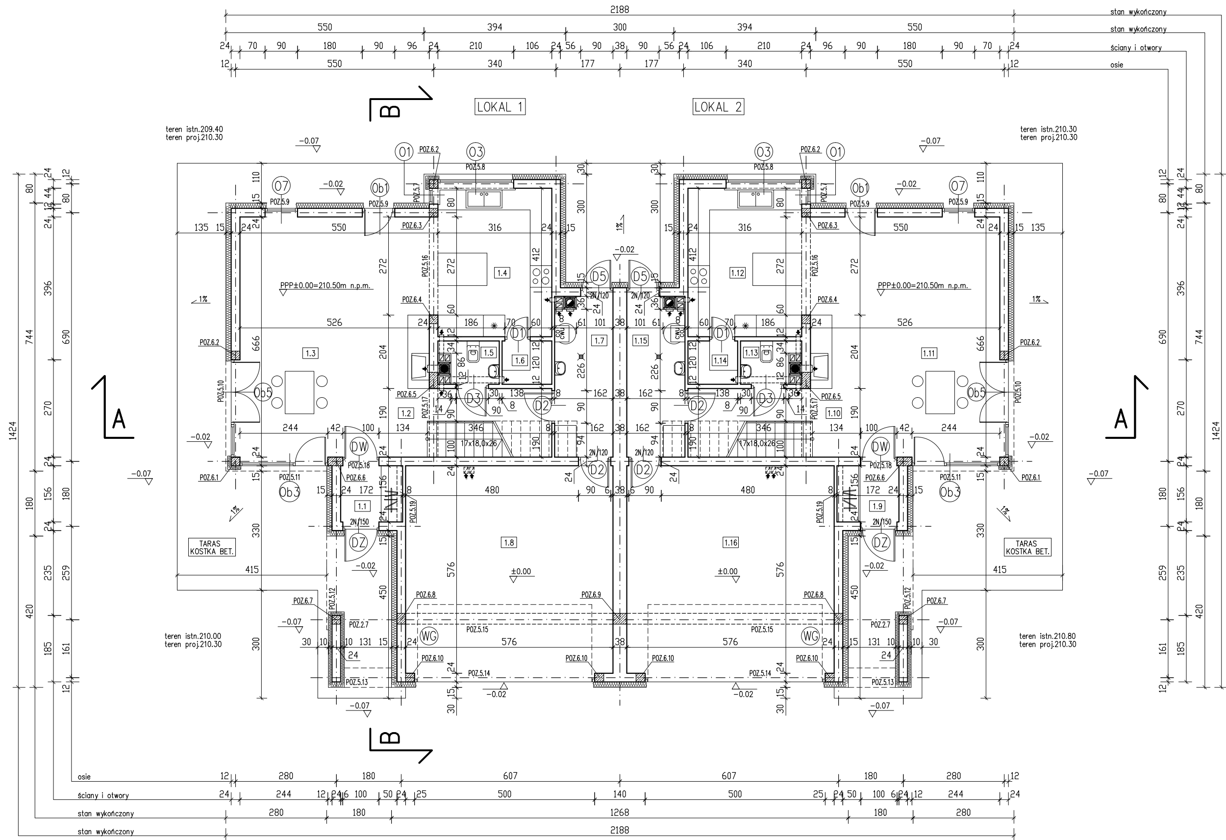
RZUT PARTERU 1:100
