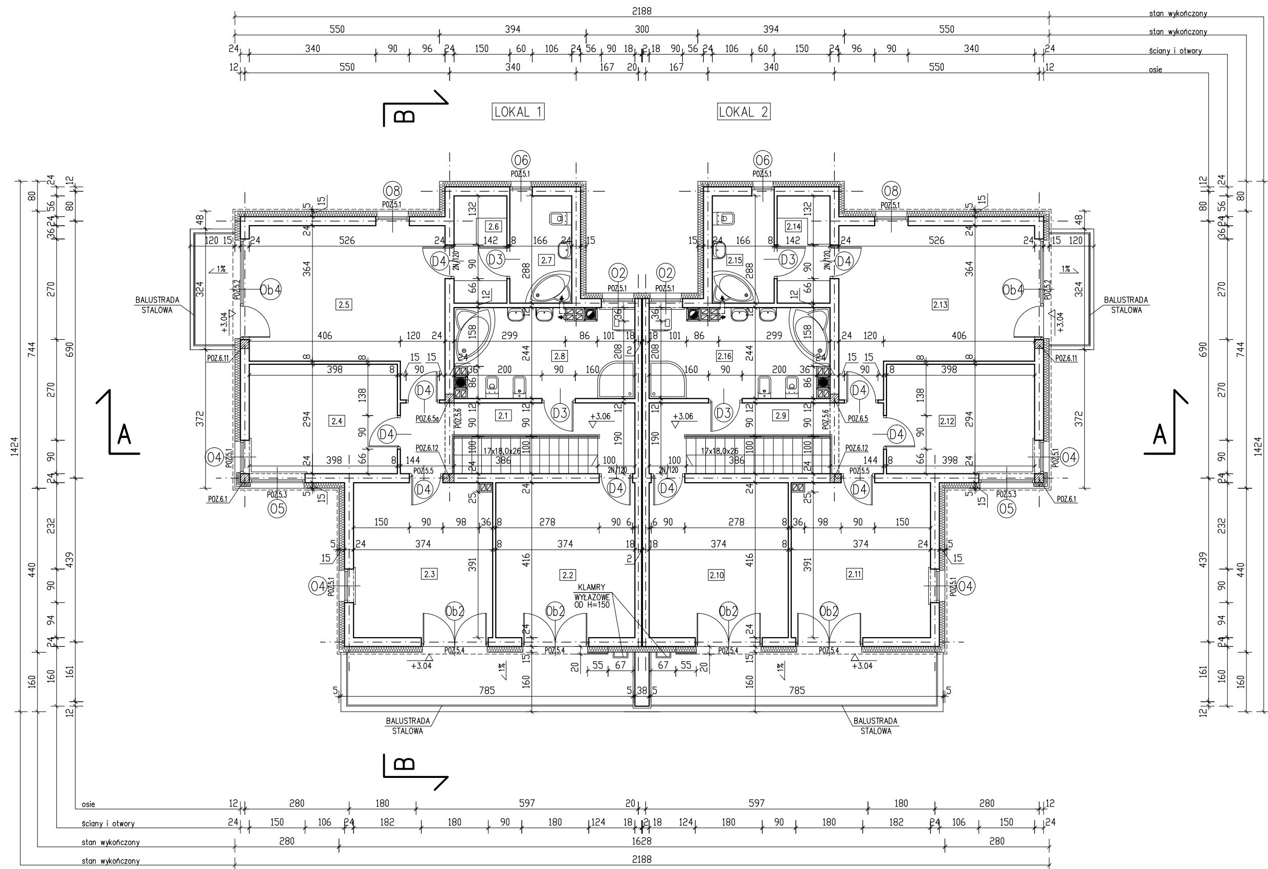
RZUT PIĘTRA 1:100
