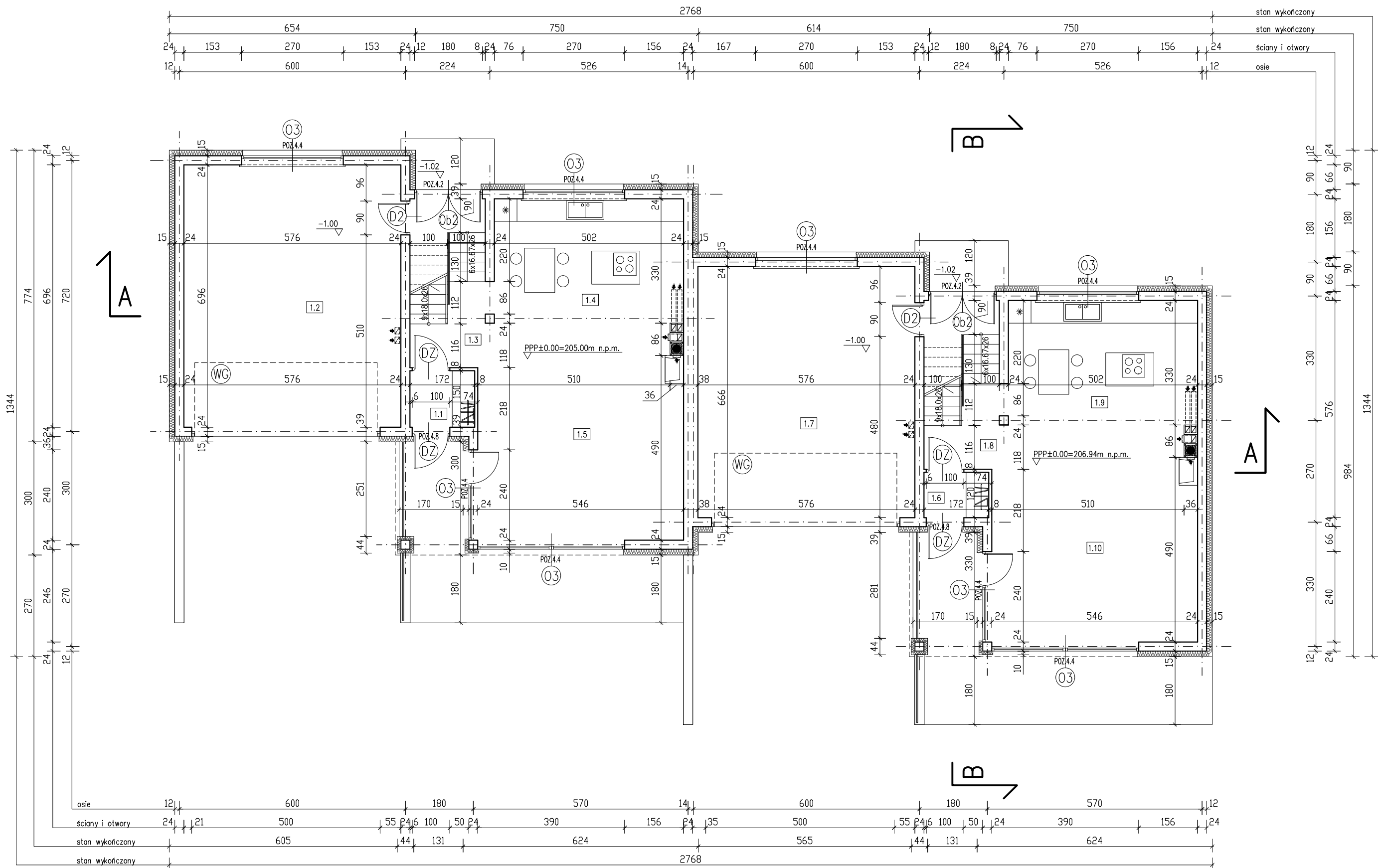
RZUT PARTERU 1:100
