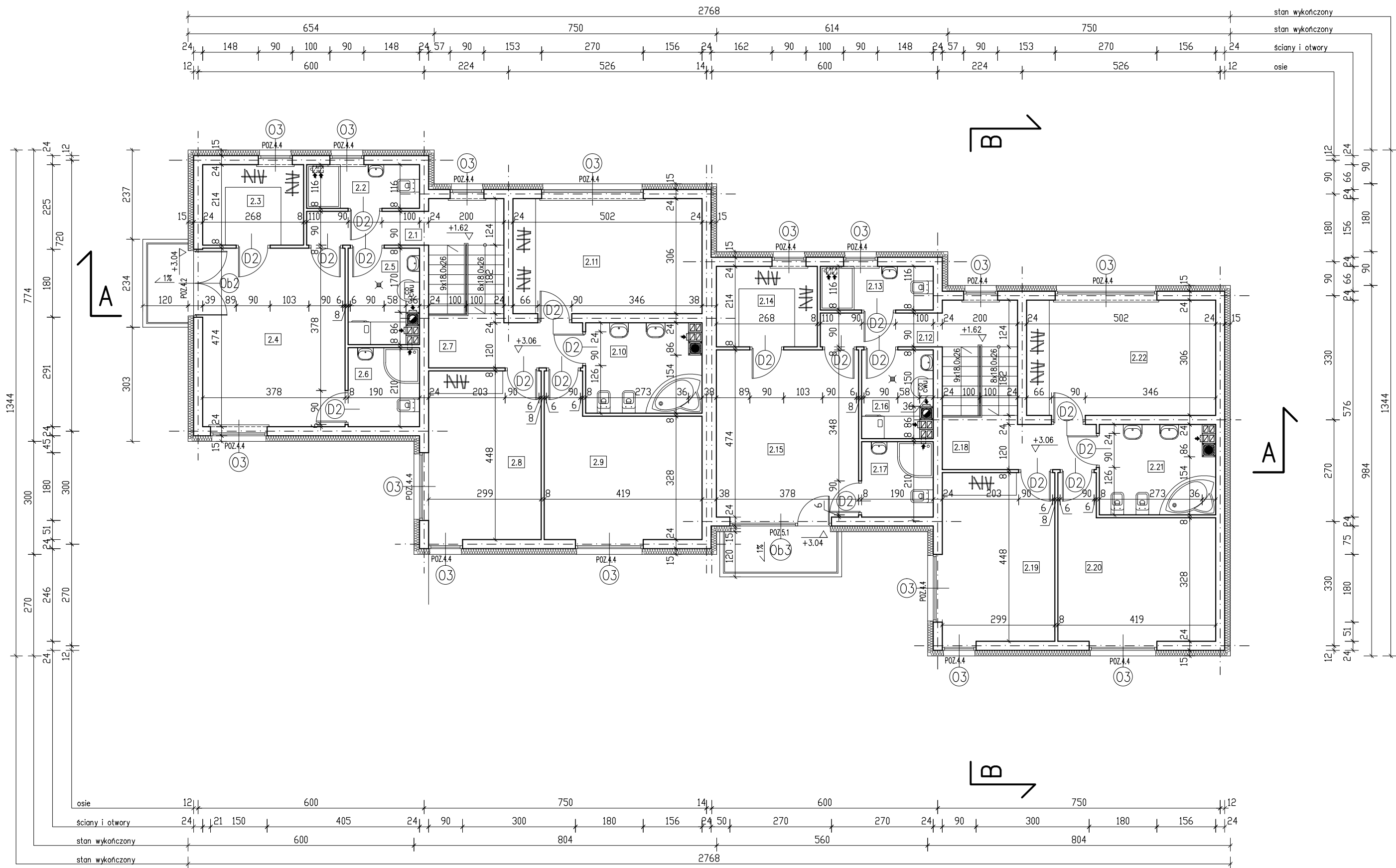
RZUT PIĘTRA 1:100
